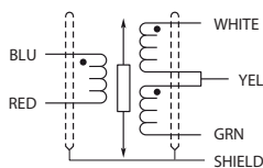
Wiring Schematic
